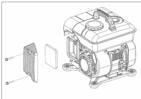
Рис. 16. Воздушный фильтр
