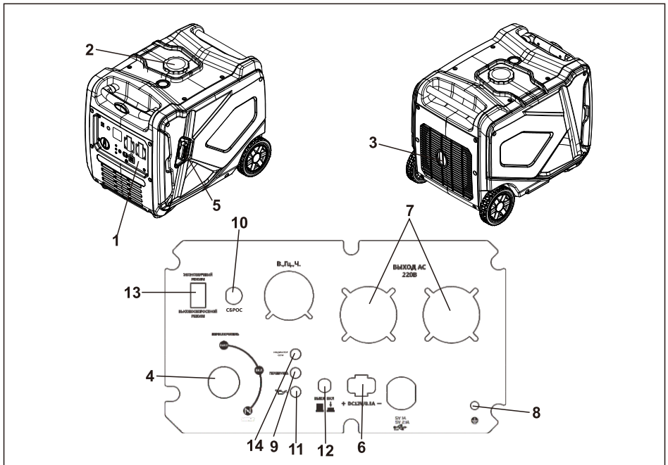
Рис.3 Общий вид модели BR5000i
