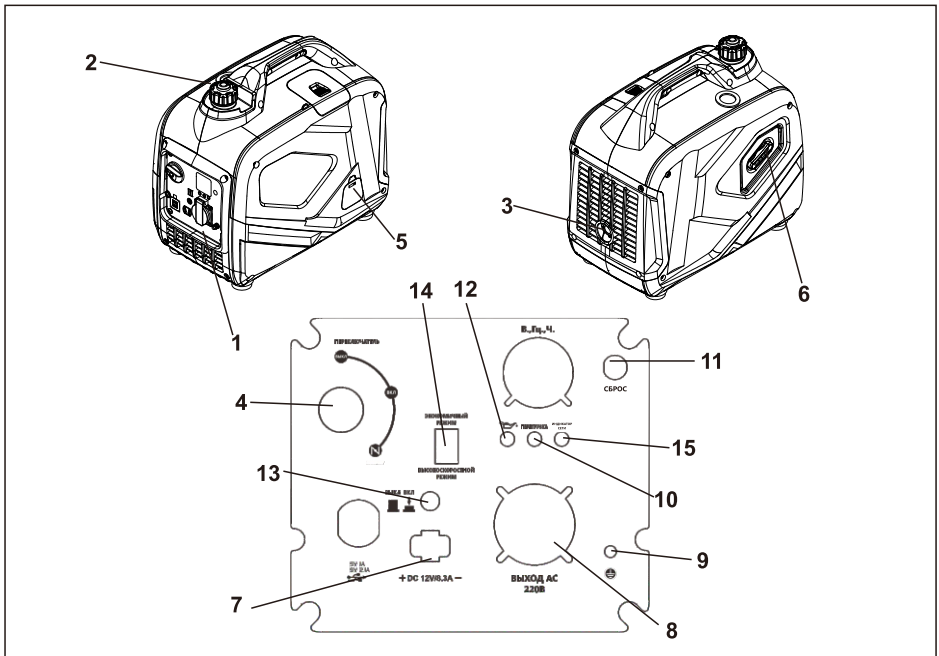
Рис.2 Общий вид модели BR3500i
