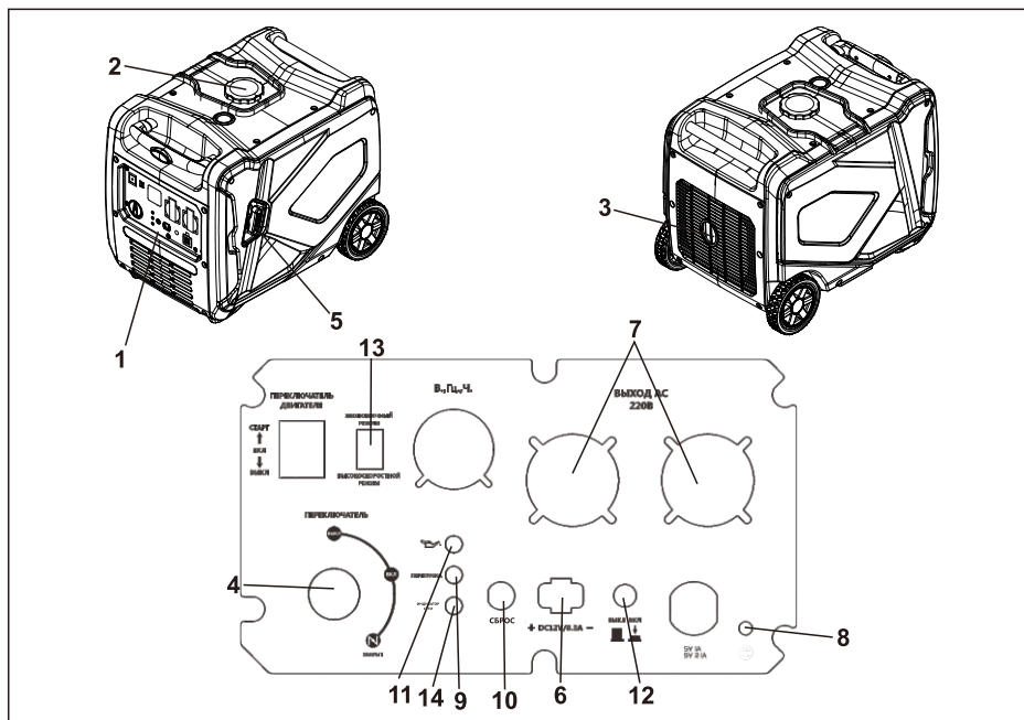
Рис.4 Общий вид модели BR7500i
